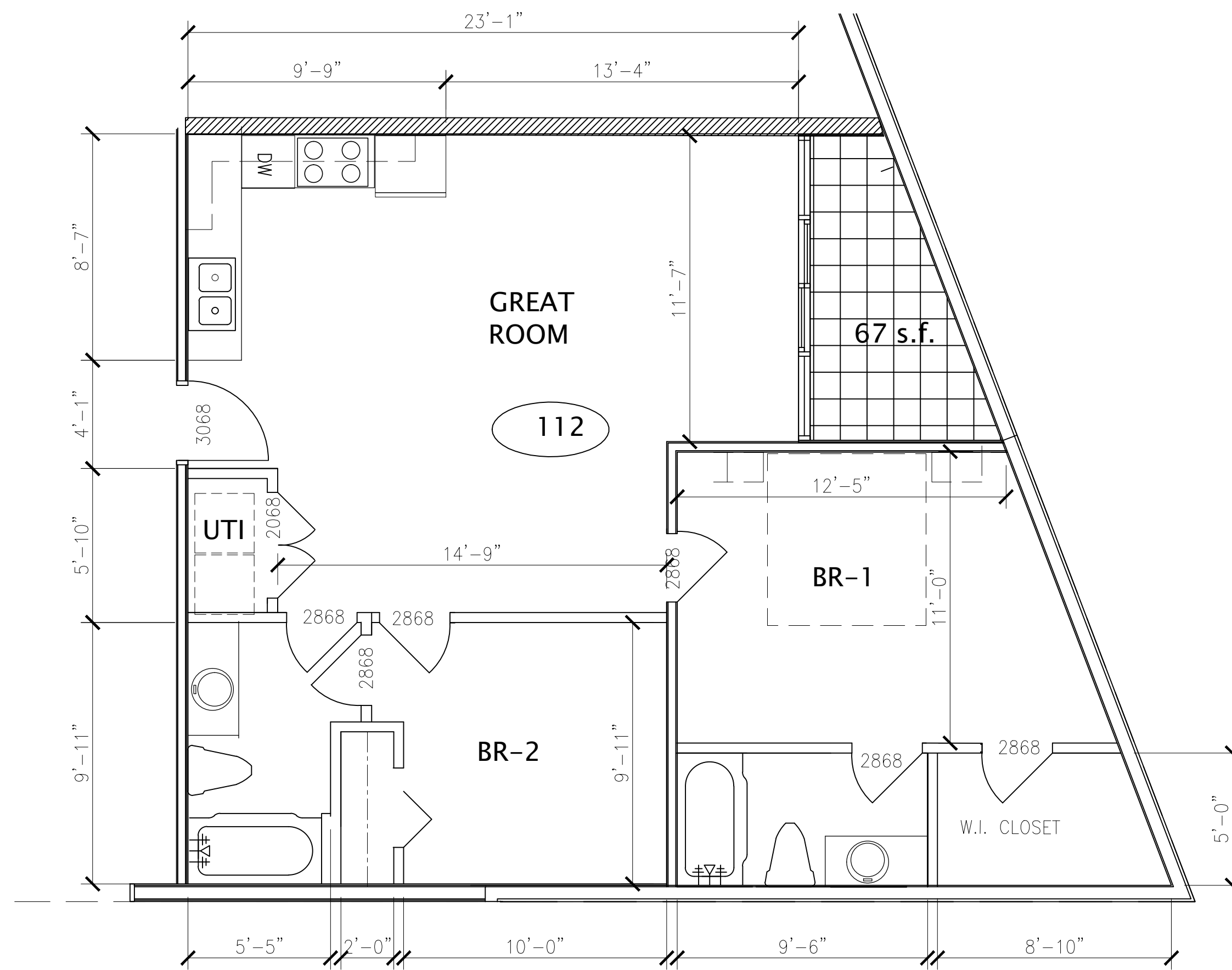
2BR-3 900 S.F.
